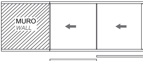
Finestra 2 ante con un'anta a scrigno Double window, with a pocket wing Fenster 2 flügel, mit einem mauerinternen flügel
